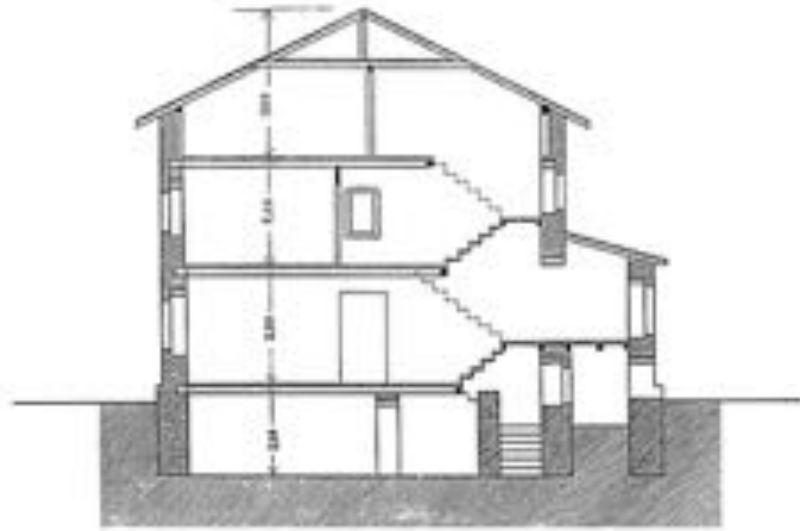
Querschnitt
